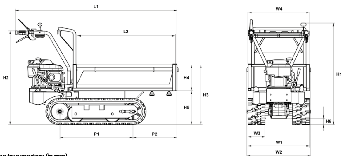
Afmetingen transporters (in mm)
