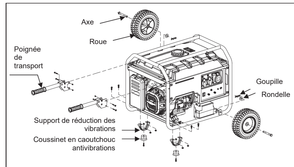
Modèle : PGE 80E-3 DCS
