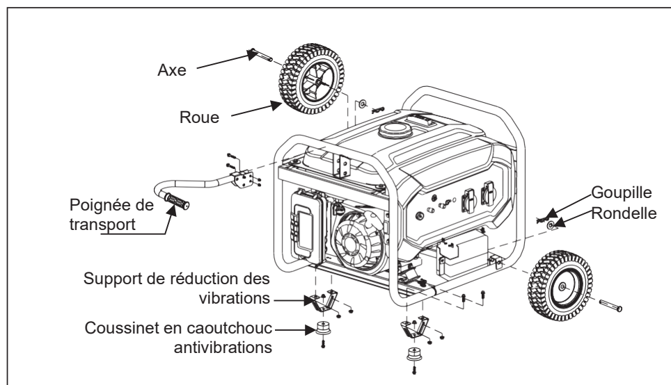
Modèle : PGE 25 DCS, PGE 35 DCS, PGE 65 DCS, PGE 65E DCS 30
